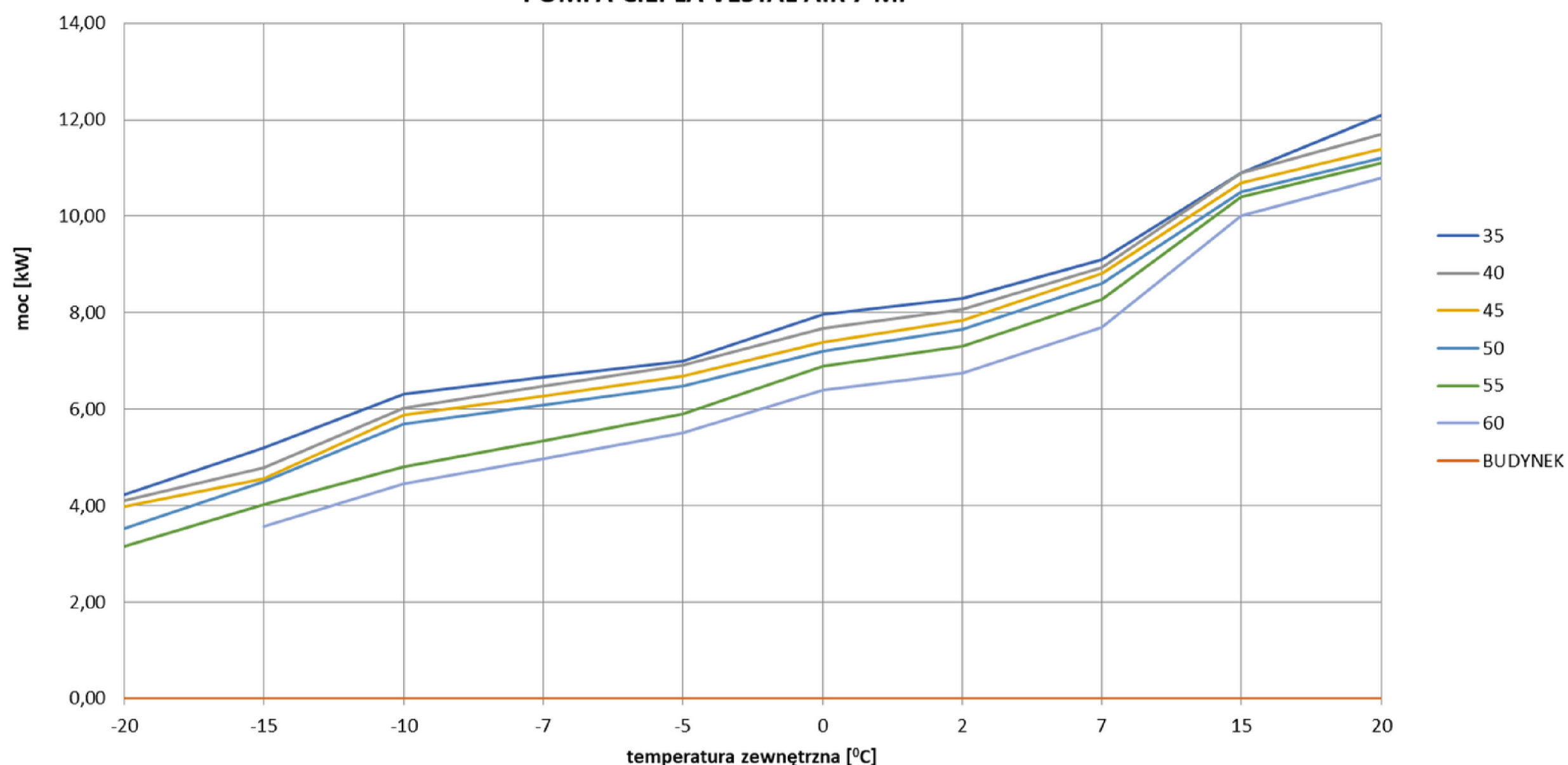
Moc pompy ciepła w zależności od temperatury zewnętrznej oraz temperatury zasilania POMPA CIEPŁA VESTAL AIR 7 MP
