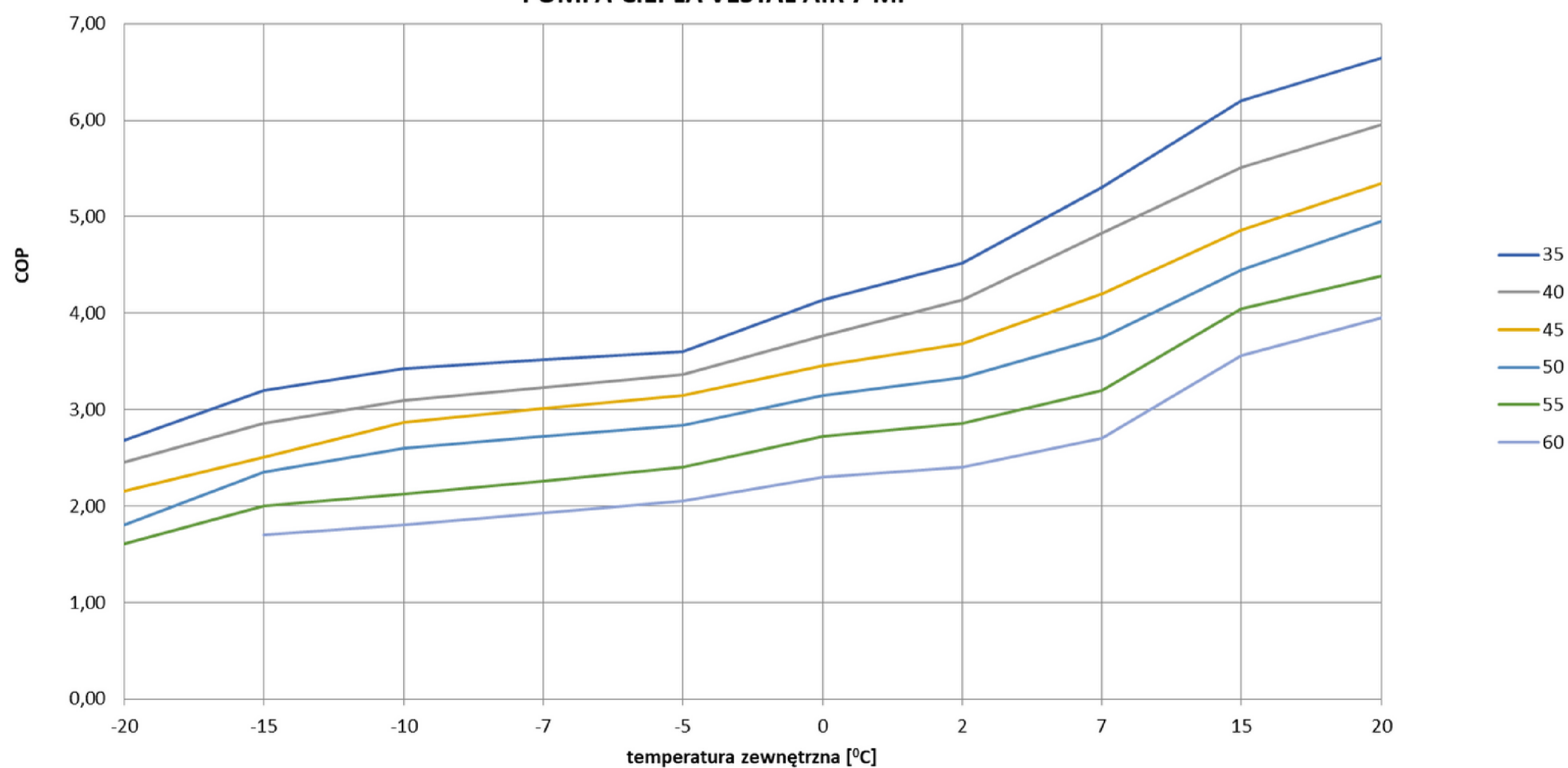
COP pompy ciepła w zależności od temperatury zewnętrznej oraz temperatury zasilania POMPA CIEPŁA VESTAL AIR 7 MP
